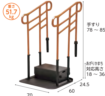
ステップ台付両手すり高さH型
