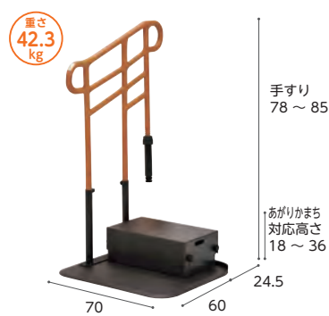
ステップ台付片手すり高さH型
