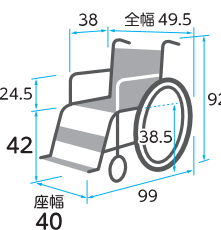
エアリー仕様 (ノーパンクタイヤ)
